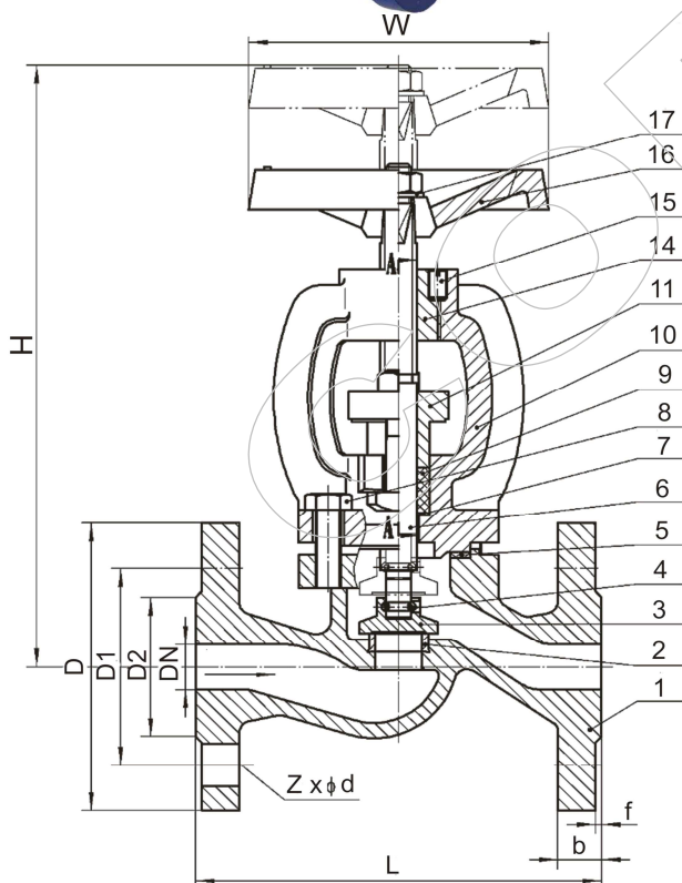
Tabulka rozměrů (mm) / Table of dimensions (mm)
