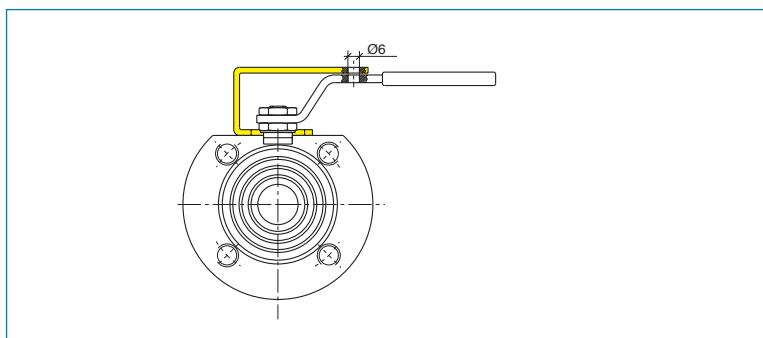
Staffa per sistema di lucchettaggio (lucchetto escluso) - Locking handle device (lockpad excluded) - Dispositif de blocage (système de cadenassage exclu) Blockiervorrichtung (Hängeschloss ausgeschlossen) - Dispositivo de bloqueo (candado no incluido)
