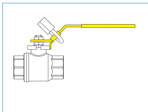
Leva per sistema di lucchettaggio (lucchetto escluso) - Locking handle device (lockpad excluded) Dispositif de blocage (système de cadenassage exclu) - Blockiervorrichtung (Hängeschloss ausgeschlossen) Dispositivo de bloqueo (candado no incluido)
