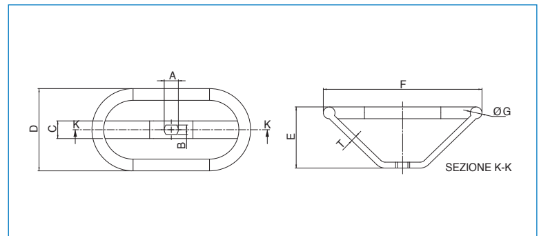
Volantino ovale per valvole flangiate e filettate - Oval handle for flanged and threaded ball valves - Oval handle pour taraudée Vanne à boisseau spérique - Oval handle für kugelhähne mit gewinde - oder flanschanschluss - Oval handle por válvula de bola roscada o bridada.
