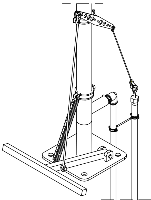
Detail: Fusshebel
