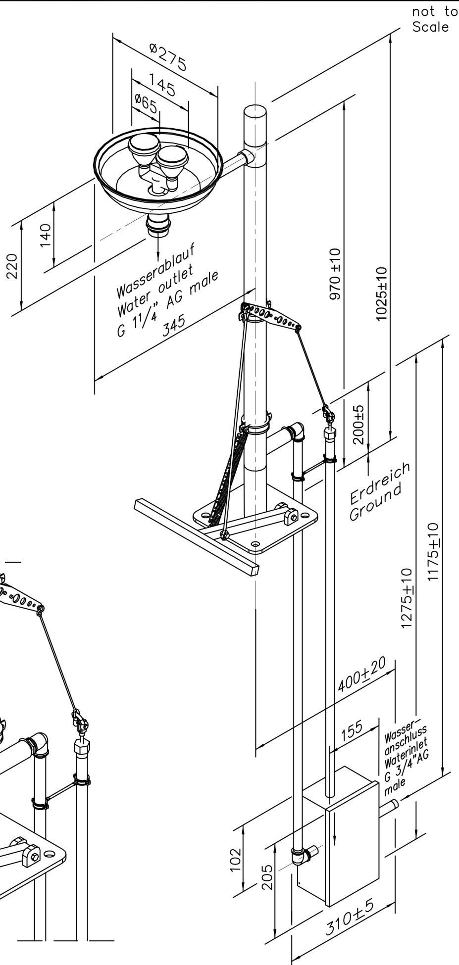
Detail: Fusshebel
