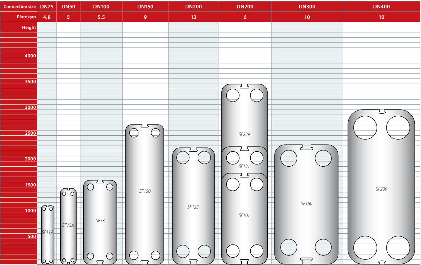
Measurements in mm Rev.11.10.2019
